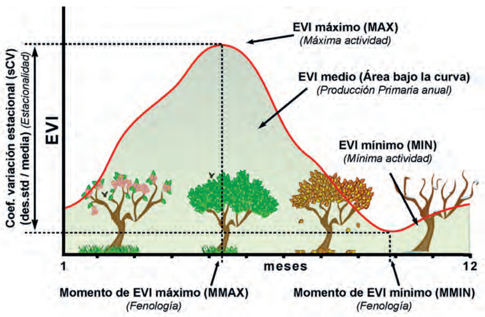
Figura 2. Curva anual de la dinámica del índice de verdor (EVI o NDVI) e indicadores del funcionamiento derivados de su parametrización.
