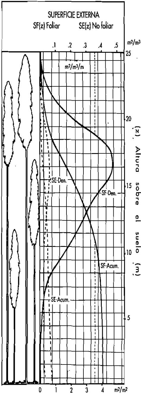
Fig. 8. Distribución vertical de la superficie externa foliar y no foliar en una plantación de Eucalyptus globulus de 14 años.
