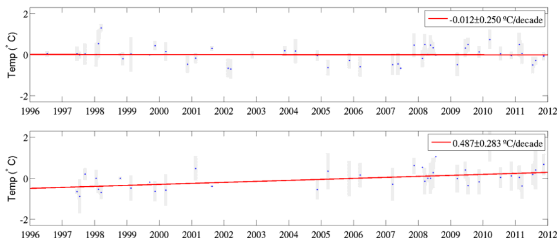
Figura 7.5. Tendencia de las anomalías de temperatura y salinidad a 150 metros (panel superior) y 400 metros (panel inferior) en la DM Sudatlántica desde 1996. Los datos provienen de la base de datos histórica actualizada con los programas actualmente en marcha en el Golfo de Cádiz. El ciclo estacional se ha retirado de la serie.
