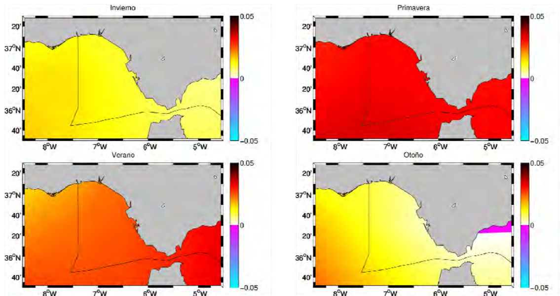
Figura 7.3. Tendencia de la SST por estaciones en la DM Sudatlántica. El registro reconstrucción SST de la NOAA (Reynolds et al. , 2002) que ofrece datos semanales en una malla de 1x1 desde principios de los 80.
