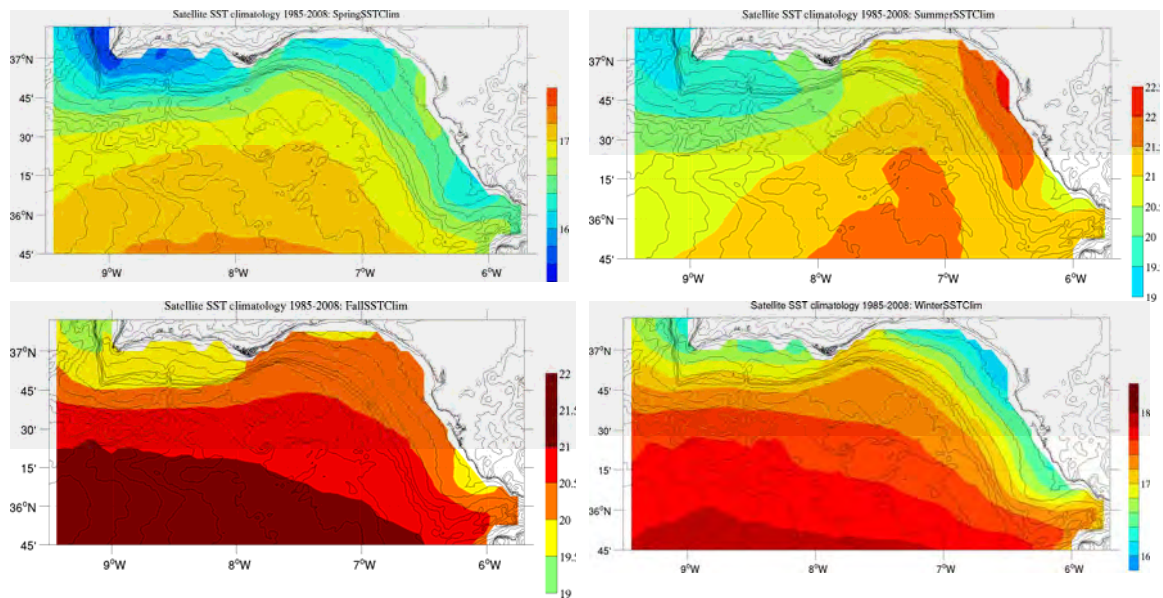
Figura 7.2. Climatología de la SST a partir de OI-SST 1985-2008.
