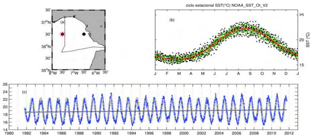
Figura 7.1. Ciclo estacional (b) y variabilidad interanual (c) de la SST en un punto representativo de la Demarcación Sudatlántica (a). El registro reconstrucción SST de la NOAA (Reynolds et al. , 2002) que ofrece datos semanales en una malla de 1x1 desde principios de los 80.
