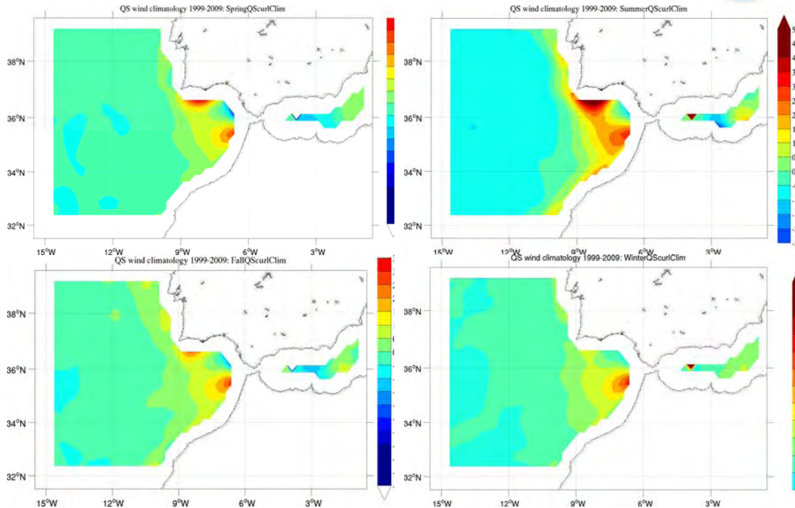
Figura 7.8. Ciclo estacional del rotacional de la tensión del viento oceánico en la región. Climatología de QuikSCAT 1999-2009.
