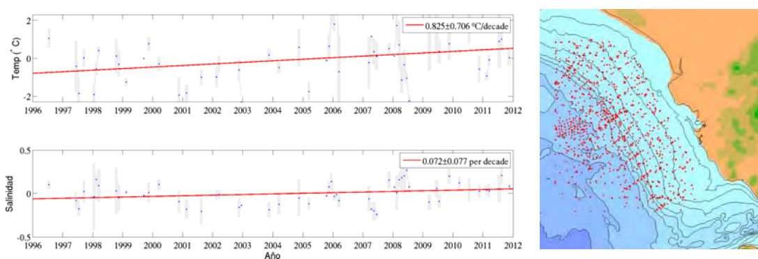
Figura 7.4. Panel izquierdo: Tendencia de las anomalías de temperatura y salinidad a 10 metros en la DM Sudatlántica desde 1996. Los datos provienen de la base de datos histórica actualizada con los programas actualmente en marcha en el Golfo de Cádiz. El ciclo estacional se ha retirado de la serie. Panel derecho: estaciones empleadas en el análisis: 1502 entre el 7 de julio de 1996 y el 24 de noviembre de 2011.
