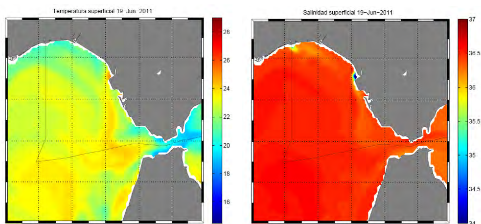
Figura 7.7b. Salidas del sistema de predicción operacional MyOcean ( www.myocean.eu ) a) SST; b) SSS.
