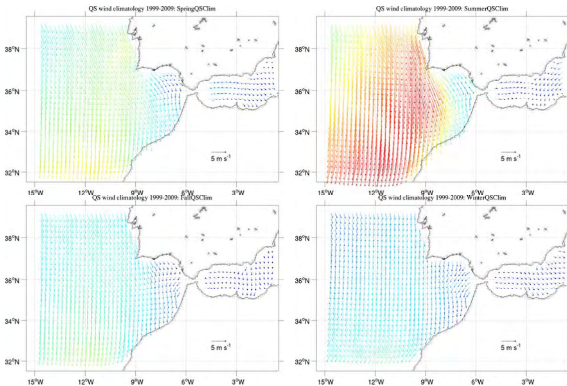
Figura 7.7. Ciclo estacional del campo de viento oceánico en la región. Climatología de QuikSCAT 1999-2009.
