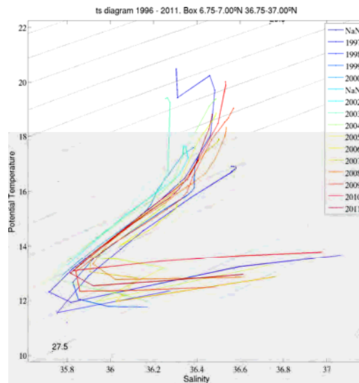
Figura 7.6. Curvas T-S obtenidas a partir de la base de datos histórica en la caja 6.75-7.00°W 36.76-37.00°N. Para 1996 y 2001 no existen datos. Para cada año, los datos se promedian a niveles estándar de NODC hasta 700 metros.
