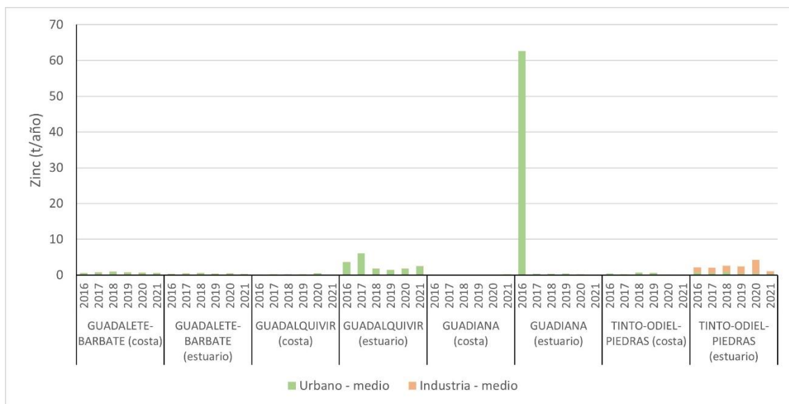
Figura 36 Aportes de zinc por vertidos directos
