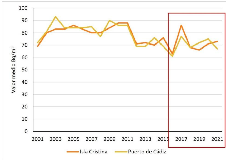
Figura 45. Concentración del índice de actividad alfa total (Bq/m 3 ) en las estaciones de la demarcación (Fuente: Figura elaborada por el CEDEX con datos publicados por el Consejo de Seguridad Nuclear)
