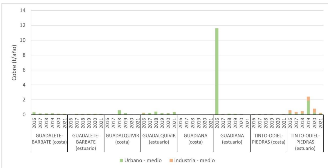
Figura 34. Aportes de cobre por vertidos directos
