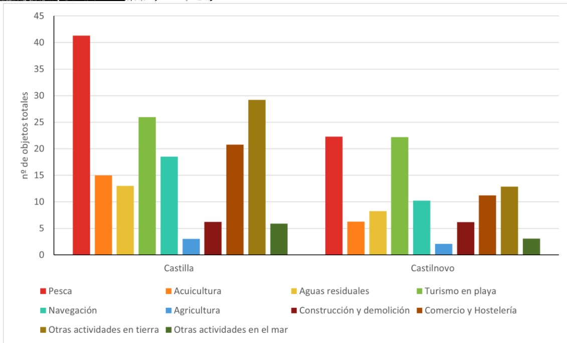
Figura 68. Distribución espacial de las fuentes de basuras marinas en las playas de la demarcación sudatlántica durante 2016-20121. (Fuente: Figura elaborada por el CEDEX a partir de datos del MITECO)
