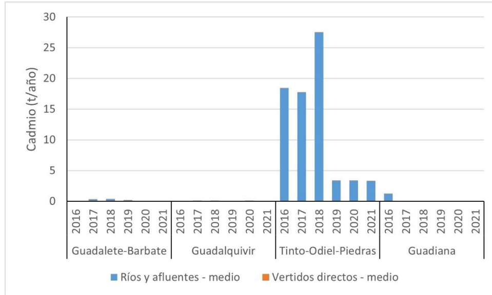
Figura 27. Aportes de cadmio desde ríos y vertidos directos
