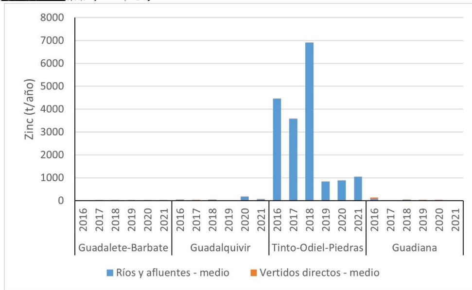
Figura 35 Aportes de zinc desde ríos y vertidos directos
