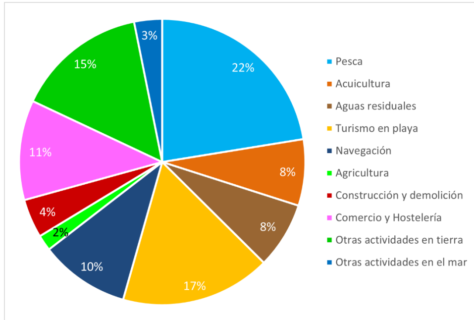
Figura 66. Fuentes de basuras marinas en las playas de la demarcación sudatlántica durante 2016-2021. (Fuente: Figura elaborada por el CEDEX a partir de datos del MITECO)
