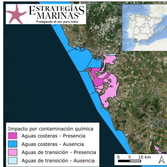
Figura 65. Masas de agua costeras y de transición impactadas por contaminación química en Cádiz
