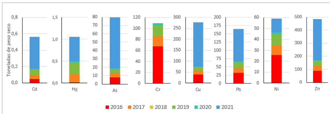
Figura 49. Aportes de metales pesados (t/año) contenidos en los sedimentos vertidos al mar procedentes de los dragados portuarios. (Fuente: Figura elaborada por el CEDEX a partir de datos del Inventario de Dragados de Puertos del Estado y de la información aportada por la capitanías marítimas y Comunidad Autónoma de Andalucía)
