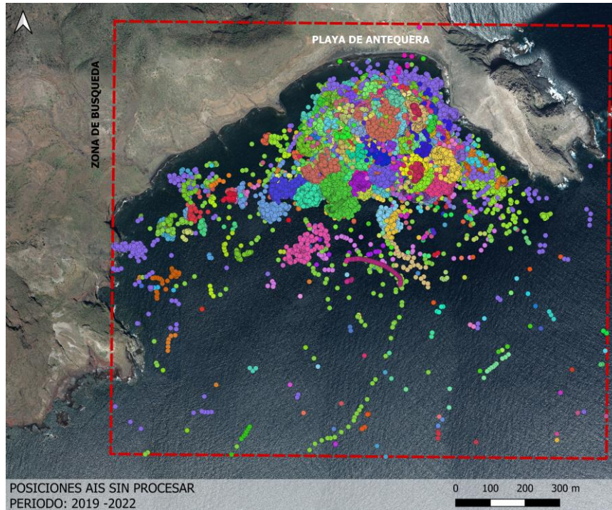
Figura 6. Posiciones AIS sin procesar (los distintos colores muestran diferentes barcos recreativos). (Fuente: Figura elaborada por el CEDEX a partir de datos AIS de SASEMAR para el proyecto europeo MSP-OR)
