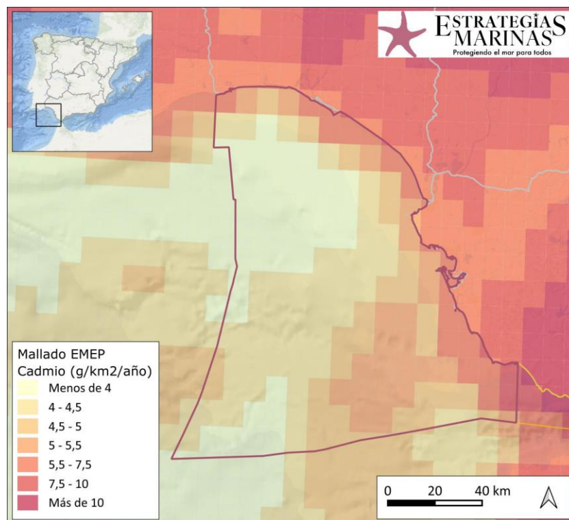
Figura 61. Masa de cadmio (Cd) depositado desde la atmósfera por unidad de superficie durante el año 2021. (Fuente: Figura elaborada por el CEDEX a partir de datos del Programa EMEP)
