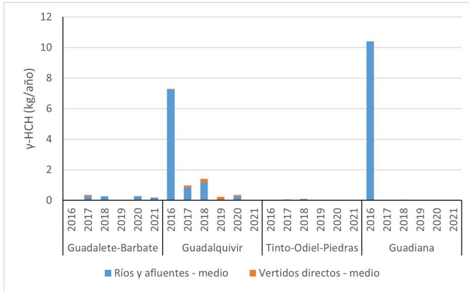
Figura 37. Aportes de \gamma -hexaclorociclohexano desde ríos y vertidos directos
