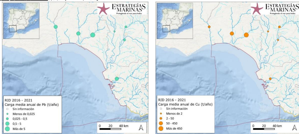
Figura 41. Carga media anual de plomo (izquierda) y cobre (derecha) aportada por ríos en el periodo 2016-2021. (Fuente: Figura elaborada por el CEDEX a partir de datos del Programa RID)
