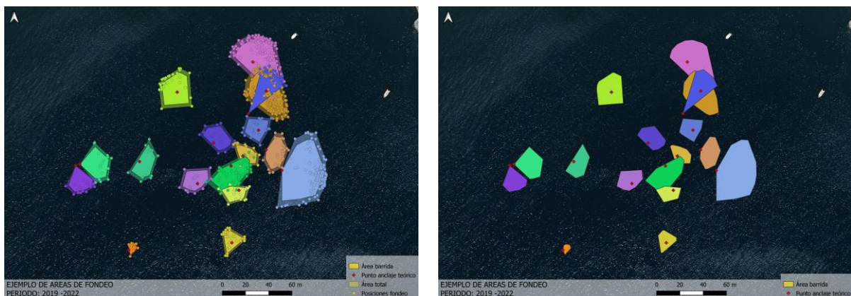
Figura 7. Posiciones AIS, envolvente y área potencialmente perturbada (los distintos colores muestran diferentes fondeos). (Fuente: Figura elaborada por el CEDEX a partir de datos AIS de SASEMAR para el proyecto europeo MSP-OR)
