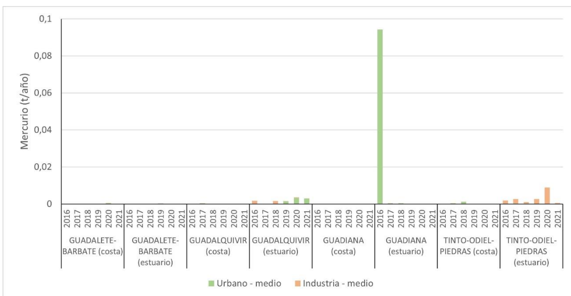
Figura 30. Aportes de mercurio por vertidos directos
