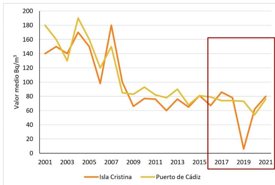
Figura 47. Concentración de actividad de tritio ( \text{Bq}/\text{m}^3 ) en las estaciones de la demarcación
