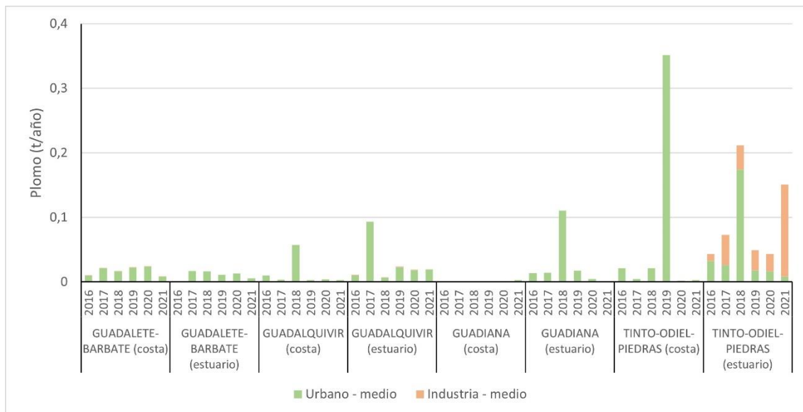
Figura 32. Aportes de plomo por vertidos directos
