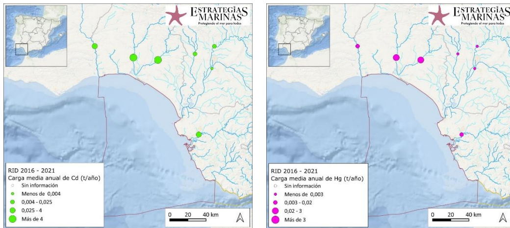
Figura 40. Carga media anual de cadmio (izquierda) y mercurio (derecha) aportada por ríos en el periodo 2016-2021. (Fuente: Figura elaborada por el CEDEX a partir de datos del Programa RID)
