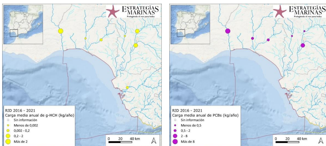
Figura 43. Carga media anual de \gamma -HCH (izquierda) y PCBs (derecha) aportada por ríos en el periodo 2016-2021. (Fuente: Figura elaborada por el CEDEX a partir de datos del Programa RID)
