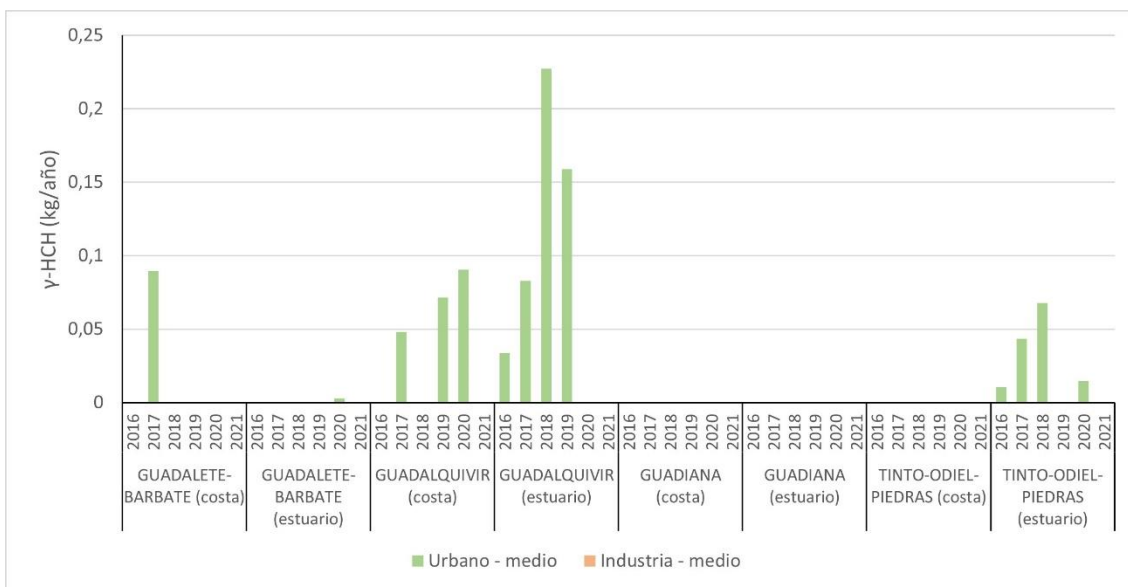
Figura 38. Aporte de \gamma -hexaclorociclohexano por vertido directos
