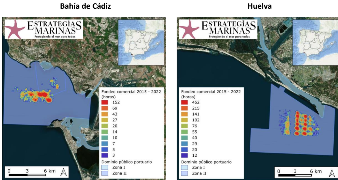
Figura 5. Horas de presencia de buques comerciales fondeados en el periodo 2015-2022. Nótese que las escalas son diferentes en cada figura. (Fuente: Figura elaborada por el CEDEX a partir de datos AIS de SASEMAR)
