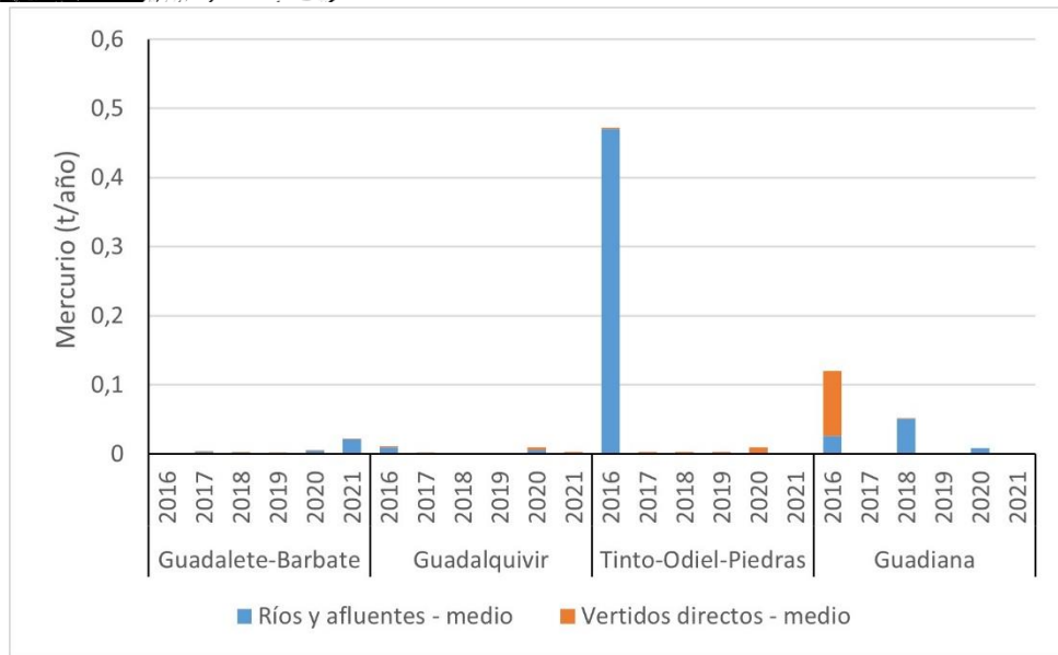
Figura 29. Aportes de mercurio desde ríos y vertidos directos
