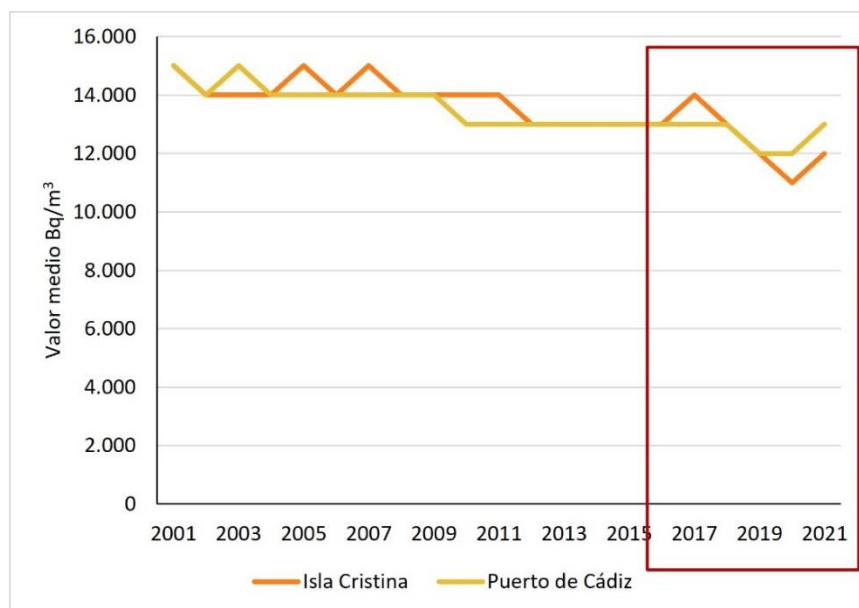
Figura 46. Concentración del índice de actividad beta total (Bq/m 3 ) en las estaciones de la demarcación (Fuente: Figura elaborada por el CEDEX con datos publicados por el Consejo de Seguridad Nuclear)
