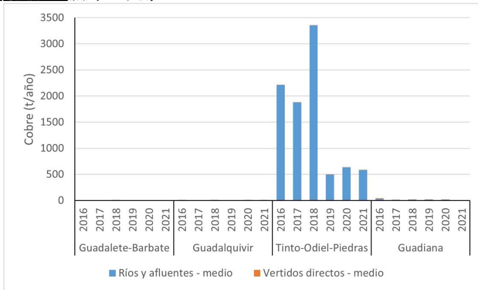
Figura 33. Aportes de cobre desde ríos y vertidos directos
