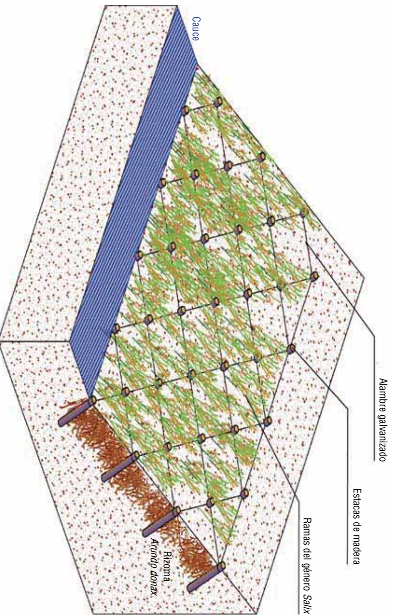
Figura 45. El método de cobertura de ramas requiere llevar a cabo una densa plantación de tallos vivos de sauce que se fijan en contacto con el sustrato. Para ello es necesario un entramado de alambres que se fijan entre estacas. Imagen: DGA (MAGRAMA) – TRAGSA.
