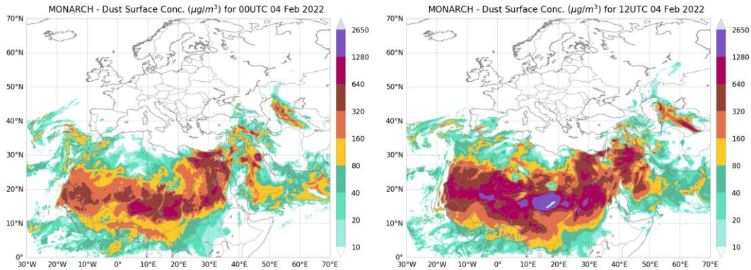
Concentración de polvo ( \mu\text{g}/\text{m}^3 ) predicha por el modelo NMMB-MONARCH para el día 4 de febrero de 2022 a las 00 y 12 UTC (izquierda y derecha, respectivamente). © Barcelona Dust Forecast Center.
