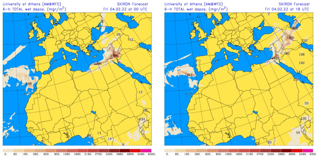
Depósito húmedo de polvo (mg/m 2 ) predicho por el modelo SKIRON para el día 4 de febrero de 2022 a las 00 y 18 UTC © Universidad de Atenas.
