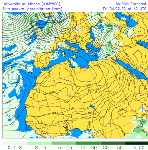
Precipitación acumulada (mm) y presión a nivel del mar (hPa) (izquierda) y campo de temperaturas (°C) y de altura geopotencial a 850 hPa (derecha) previsto por el modelo SKIRON para el día 4 de febrero de 2022 a las 12 UTC © Universidad de Atenas.
