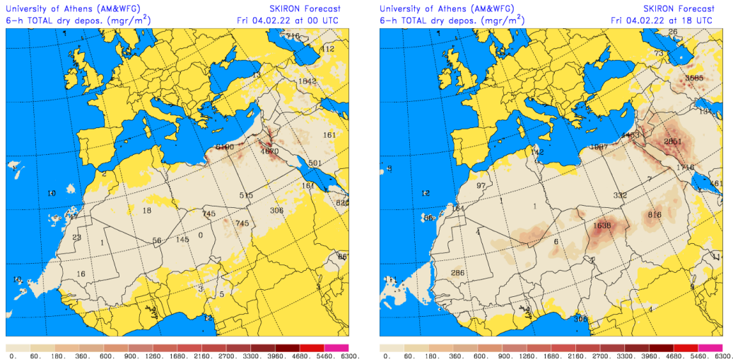
Depósito seco de polvo (mg/m 2 ) predicho por el modelo SKIRON para el día 4 de febrero de 2022 a las 00 y 18 UTC © Universidad de Atenas.
