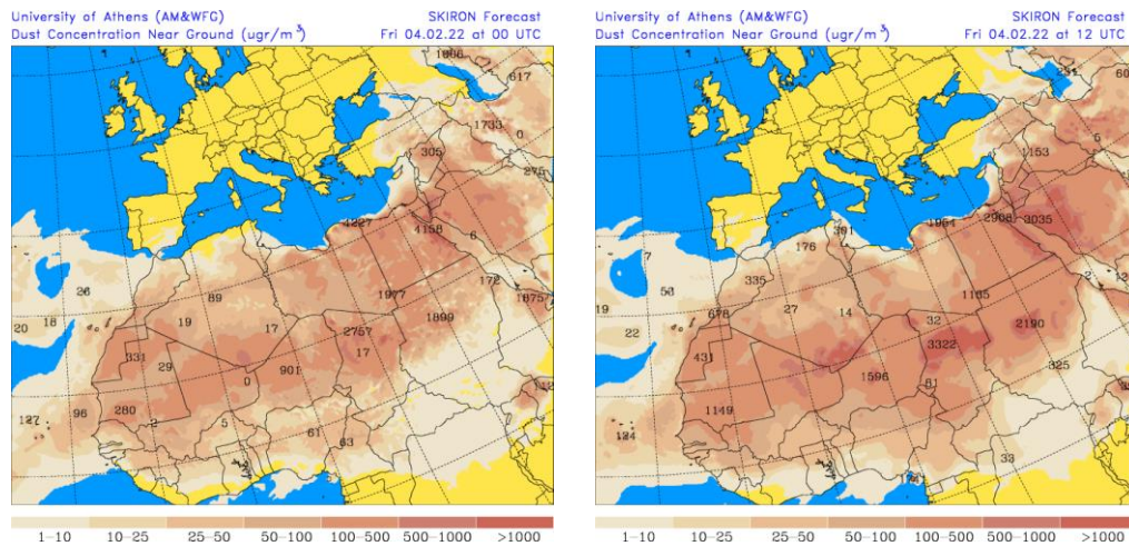
Concentración de polvo ( \mu\text{g}/\text{m}^3 ) predicha por el modelo SKIRON para el día 4 de febrero de 2022 a las 00 y 12 UTC © Universidad de Atenas.
