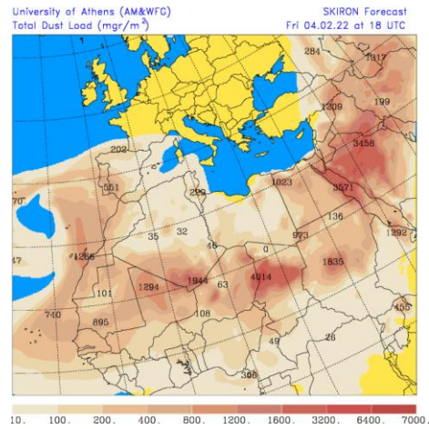
Carga total de polvo (mg/m 2 ) predicha por el modelo SKIRON para el día 4 de febrero de 2022 a las 00 y 18 UTC © Universidad de Atenas.
