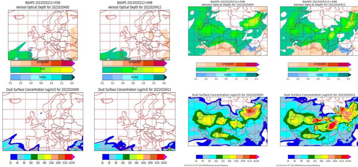
Espesor óptico de aerosoles a 550 nm (arriba) y concentración de polvo a nivel de superficie (abajo) previstos por el modelo NAAPS para el día 4 de febrero de 2022 a las 00 h UTC y a las 12 h UTC. ©Naval Research Laboratory (NRL), Monterey, CA.
