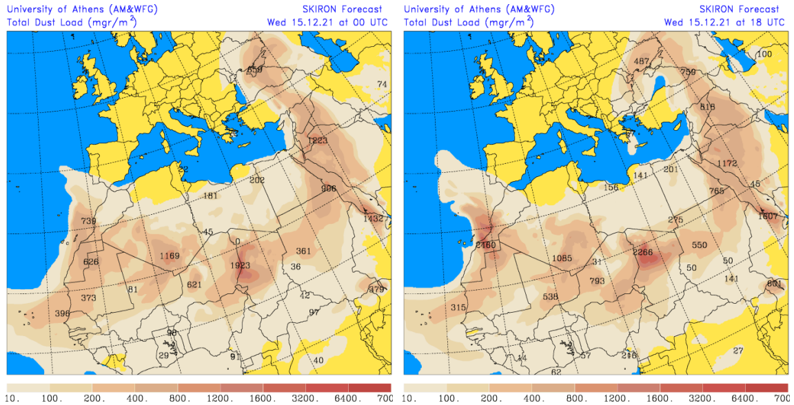
Carga total de polvo (mg/m 2 ) predicha por el modelo SKIRON para el día 15 de diciembre de 2021 a las 00 y 18 UTC © Universidad de Atenas.
