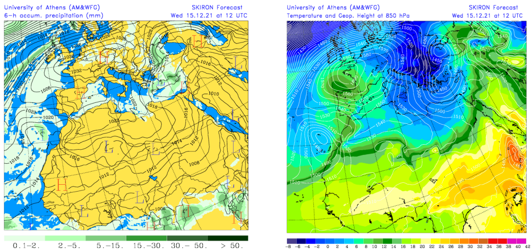
Precipitación acumulada (mm) y presión a nivel del mar (hPa) (izquierda) y campo de temperaturas (°C) y de altura geopotencial a 850 hPa (derecha) previsto por el modelo SKIRON para el día 15 de diciembre de 2021 a las 12 UTC © Universidad de Atenas.
