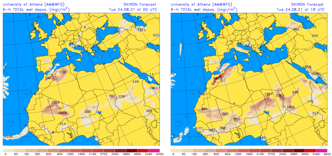
Depósito húmedo de polvo (mg/m 2 ) predicho por el modelo Skiron para el día 24 de agosto de 2021 a las 00 (izquierda) y a las 18 UTC (derecha). © Universidad de Atenas.
