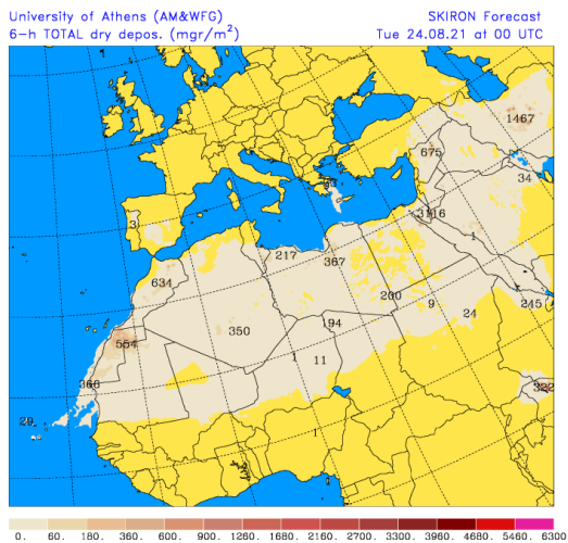
Depósito seco de polvo (mg/m 2 ) predicho por el modelo Skiron para el día 24 de agosto de 2021 a las 00 (izquierda) y a las 18 UTC (derecha). © Universidad de Atenas.
