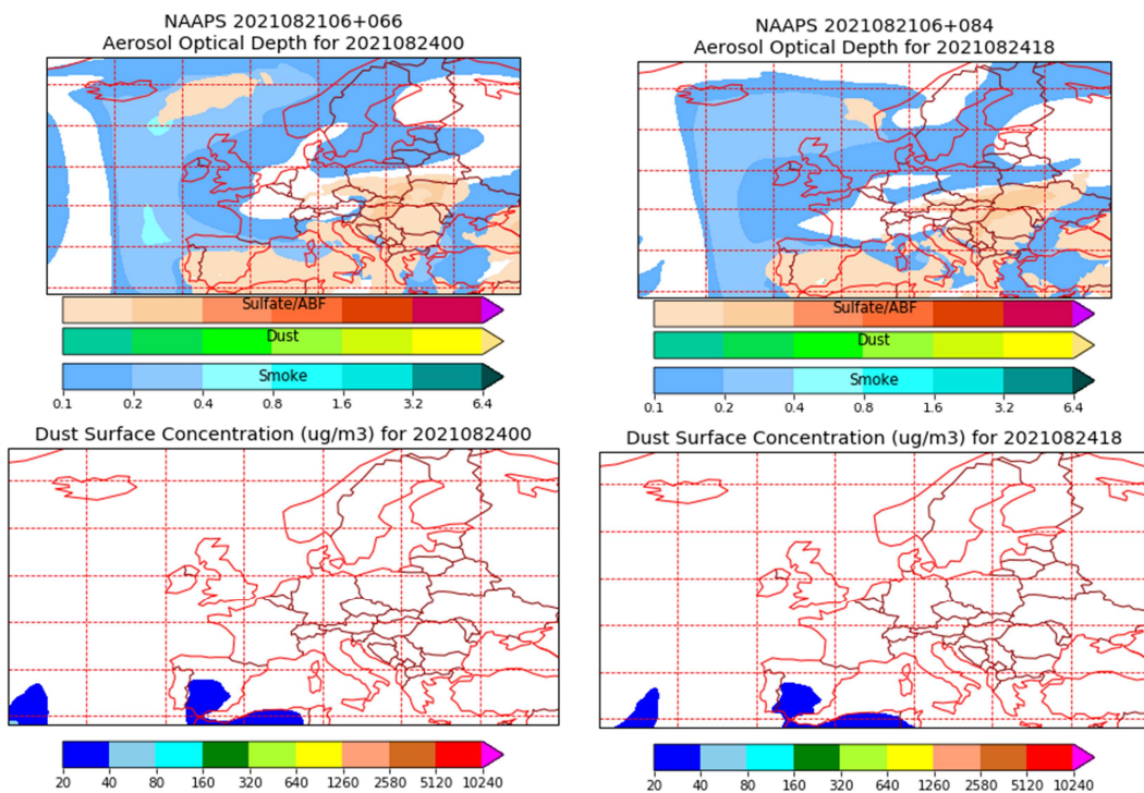
Espesor óptico de aerosoles a 550 nm (arriba) y concentración de polvo a nivel de superficie (abajo) previstos por el modelo NAAPS para el día 24 de agosto de 2021 a las 00 (izquierda) y a las 18 (derecha) UTC en Europa. ©Naval Research Laboratory (NRL), Monterey, CA
