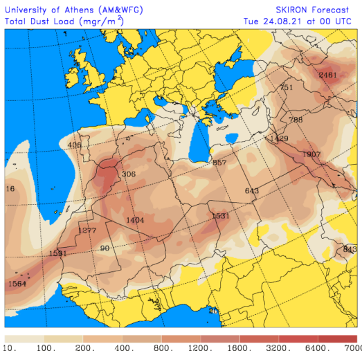
Carga total de polvo (mgr/m 2 ) predicha por el modelo Skiron para el día 24 de agosto de 2021 a las 00 (izquierda) y a las 18 UTC (derecha). © Universidad de Atenas.
