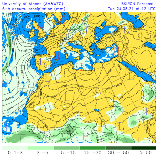
Campo de presión a nivel del mar (mb) y de precipitación (mm) (izquierda) y de temperaturas (°C) y de altura de geopotencial (m) a 850 hPa (derecha) previsto por el modelo Skiron para el día 24 de agosto de 2021 a las 12 UTC. © Universidad de Atenas.
