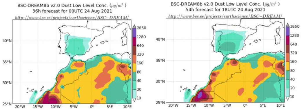
Concentración de polvo ( \mu\text{g}/\text{m}^3 ) predicha por el modelo BSC-DREAM8b v2.0 para el día 24 de agosto de 2021 a las 00 (izquierda) y a las 18 UTC (derecha). © Barcelona Supercomputing Center.
