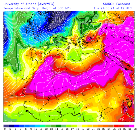
Campo de presión a nivel del mar (mb) y de precipitación (mm) (izquierda) y de temperaturas (°C) y de altura de geopotencial (m) a 850 hPa (derecha) previsto por el modelo Skiron para el día 24 de agosto de 2021 a las 12 UTC. © Universidad de Atenas.
