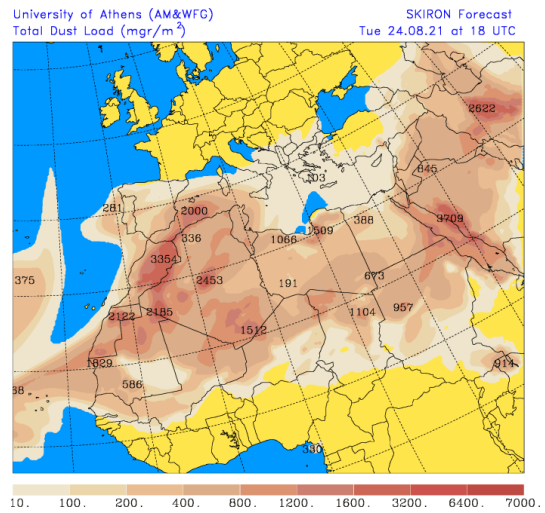
Carga total de polvo (mgr/m 2 ) predicha por el modelo Skiron para el día 24 de agosto de 2021 a las 00 (izquierda) y a las 18 UTC (derecha). © Universidad de Atenas.
