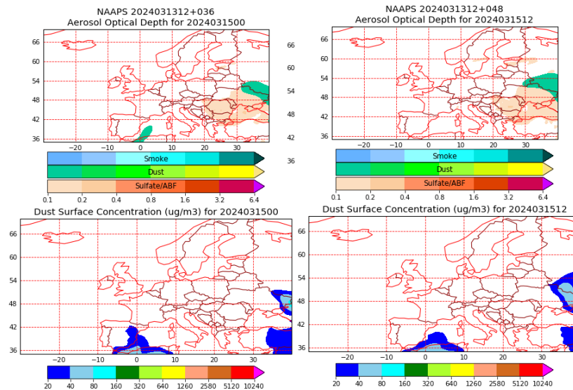
Espesor óptico de aerosoles a 550 nm (arriba) y concentración de polvo a nivel de superficie (abajo) previstos por el modelo NAAPs para el día 15 de marzo de 2024 a las 00 h UTC y a las 12 h UTC. ©Naval Research Laboratory (NRL), Monterey, CA.
