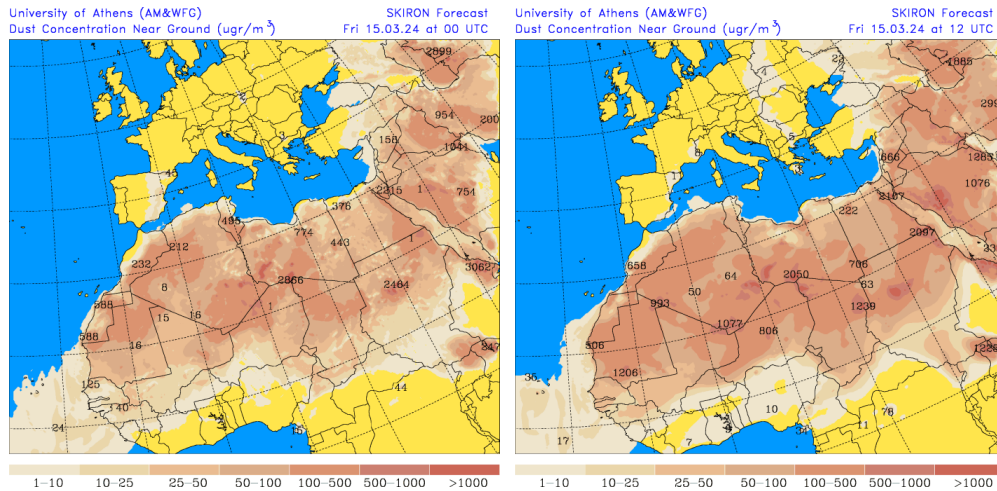
Concentración de polvo ( \mu\text{g}/\text{m}^3 ) predicha por el modelo SKIRON para el día 15 de marzo de 2024 a las 00 y 12 UTC © Universidad de Atenas.
