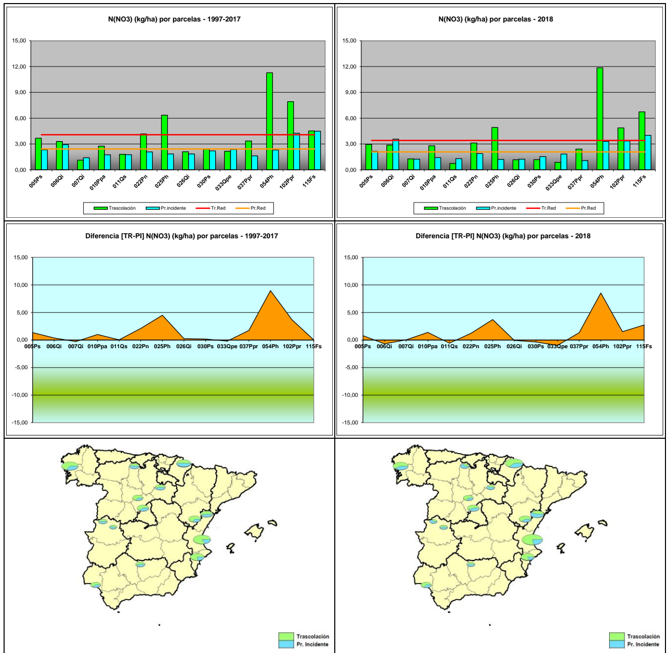
FIG 22: Deposición nitratos (kg/ha). Valores medios por parcela y diferencia entre trascolación y precipitación a campo abierto serie histórica 1997-2017 y año 2018
