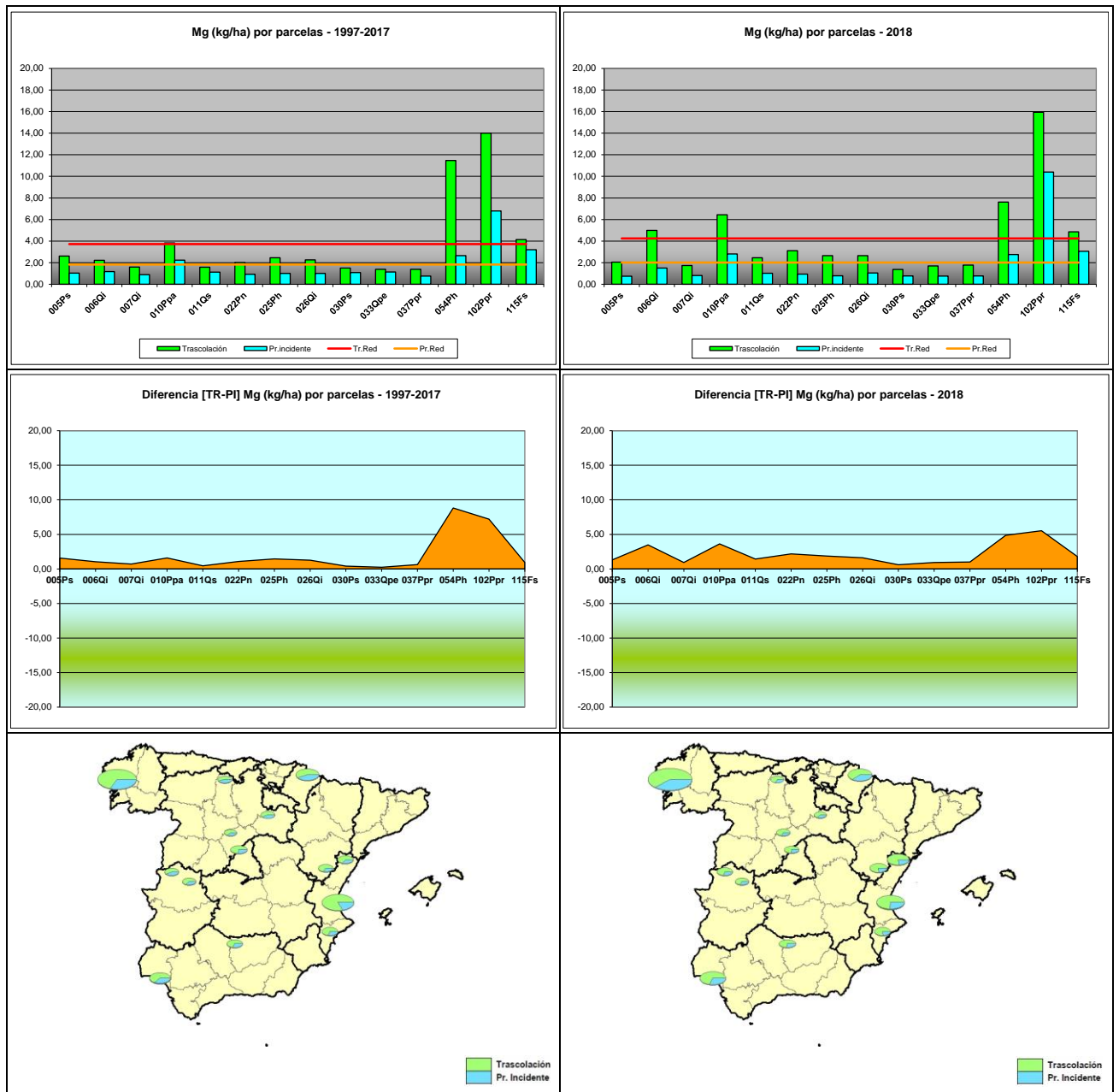
FIG 18: Deposición magnesio (kg/ha). Valores medios por parcela y diferencia entre trascolución y precipitación a campo abierto serie histórica 1997-2017 y año 2018
