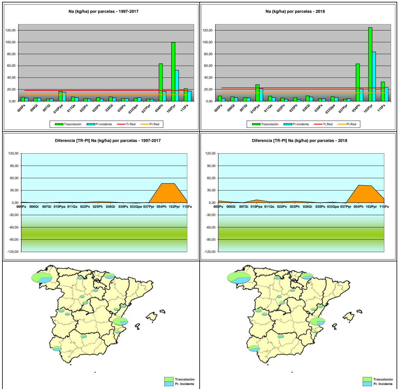
FIG 19: Deposición sodio (kg/ha). Valores medios por parcela y diferencia entre trascolación y precipitación a campo abierto serie histórica 1997-2017 y año 2018
