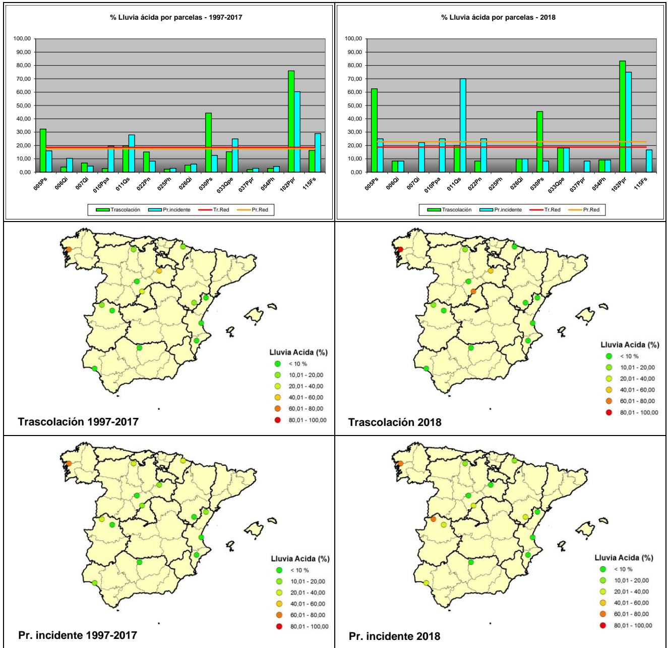
FIG 14: pH. Valores medios por parcela y porcentaje de precipitaciones por debajo del umbral de lluvia ácida serie histórica 1997-2017 y año 2018
