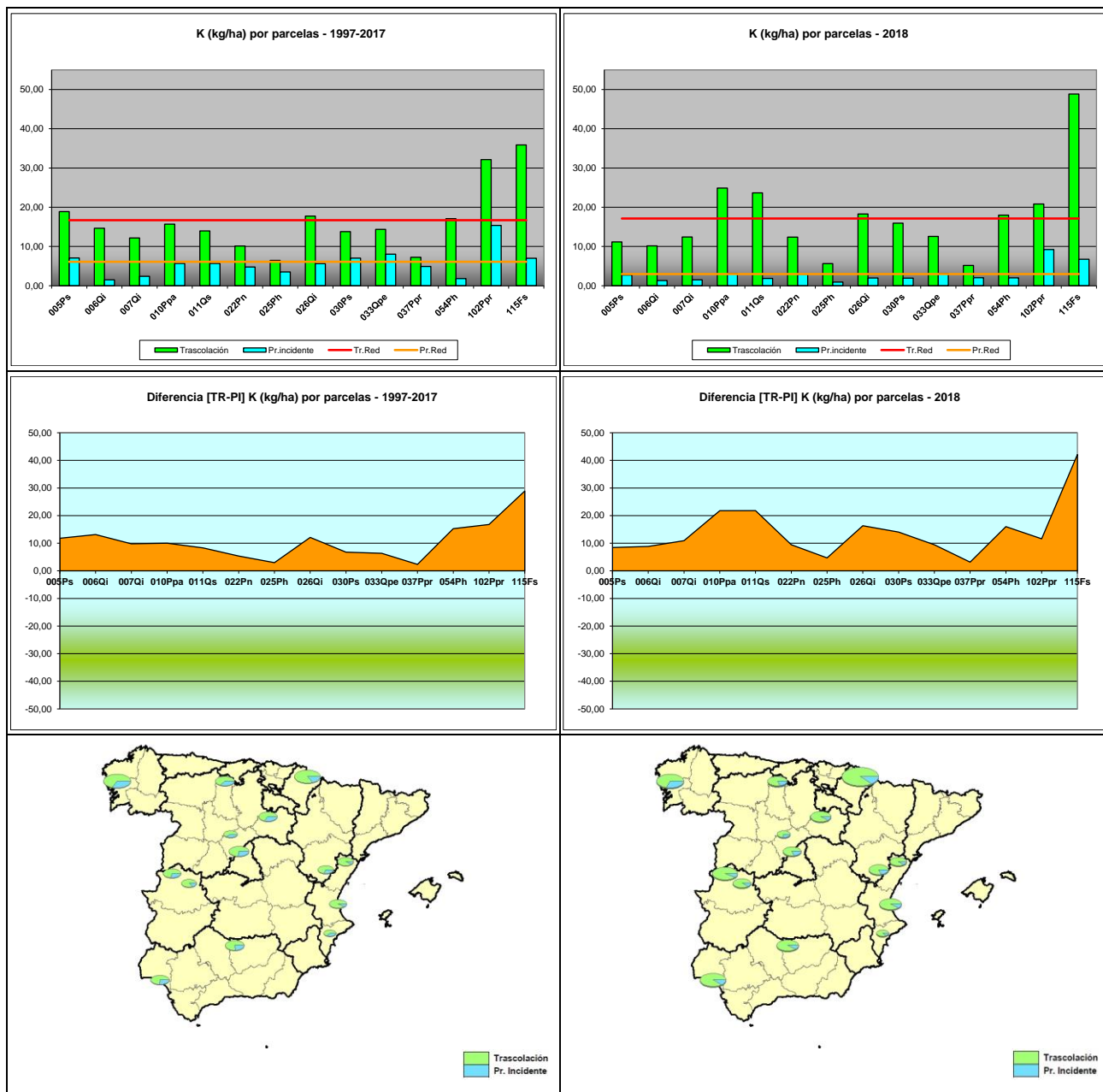
FIG 16: Deposition potasio (kg/ha). Valores medios por parcela y diferencia entre trascolación y precipitación a campo abierto serie histórica 1997-2017 y año 2018
