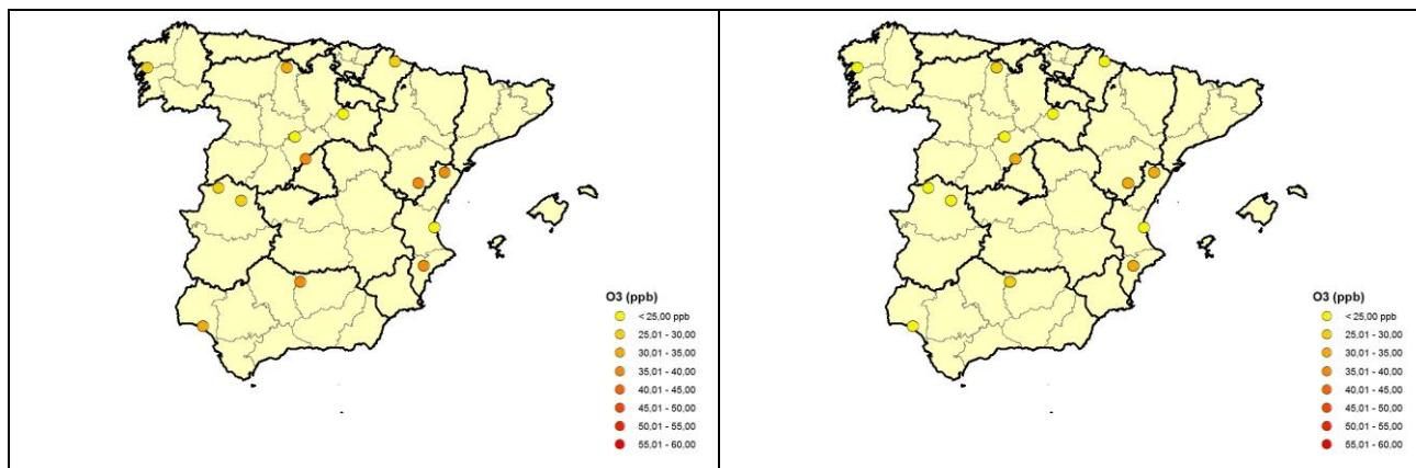
FIG 24: Inmisión atmosférica. Dióxido de azufre, óxidos de nitrógeno, amoníaco y ozono. Valores medios por parcela serie histórica 2000-2018 y año 2019
