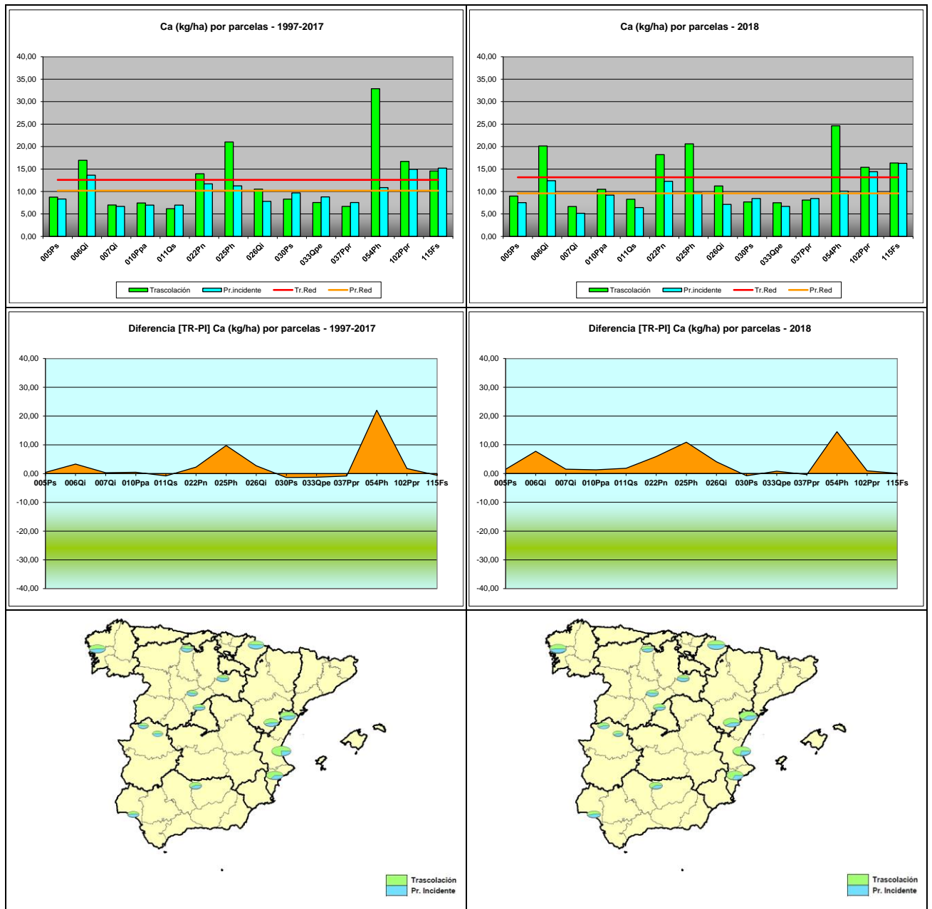
FIG 17: Deposición calcio (kg/ha). Valores medios por parcela y diferencia entre trascolación y precipitación a campo abierto serie histórica 1997-2017 y año 2018
