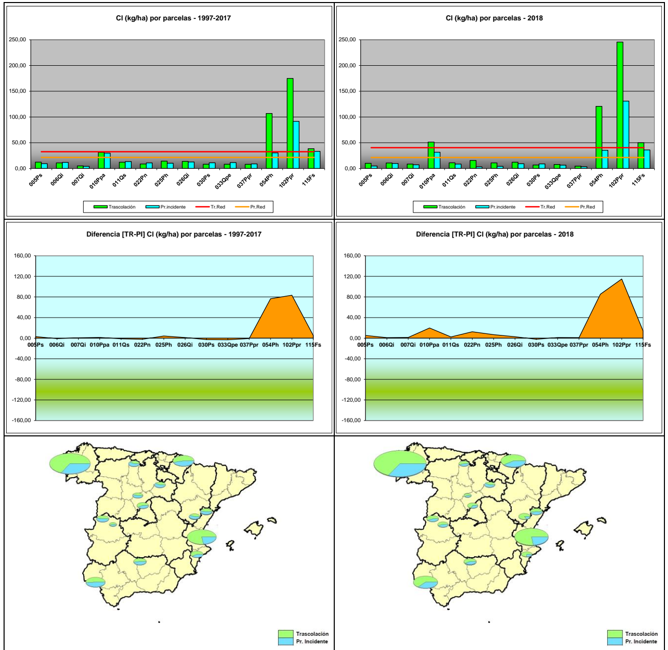
FIG 21: Deposición cloro (kg/ha). Valores medios por parcela y diferencia entre traslación y precipitación a campo abierto serie histórica 1997-2017 y año 2018
