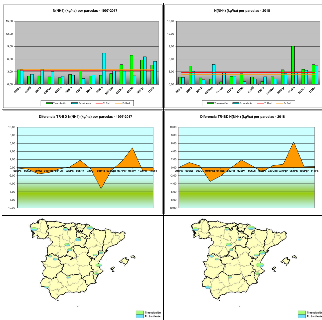
FIG 20: Deposición amonio (kg/ha). Valores medios por parcela y diferencia entre trascolución y precipitación a campo abierto serie histórica 1997-2017 y año 2018
