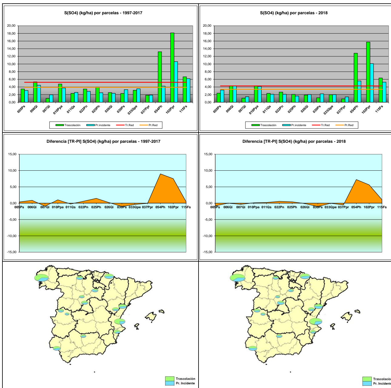
FIG 23: Deposición sulfatos (kg/ha). Valores medios por parcela y diferencia entre trascolución y precipitación a campo abierto serie histórica 1997-2017 y año 2018
