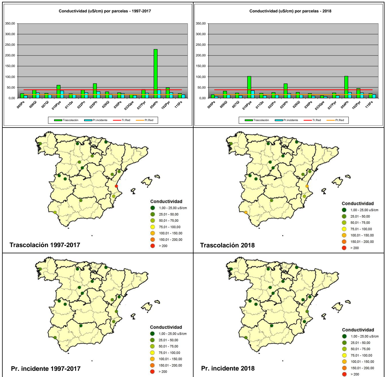
FIG 15: Conductividad. Valores medios por parcela serie histórica 1997-2017 y año 2018
