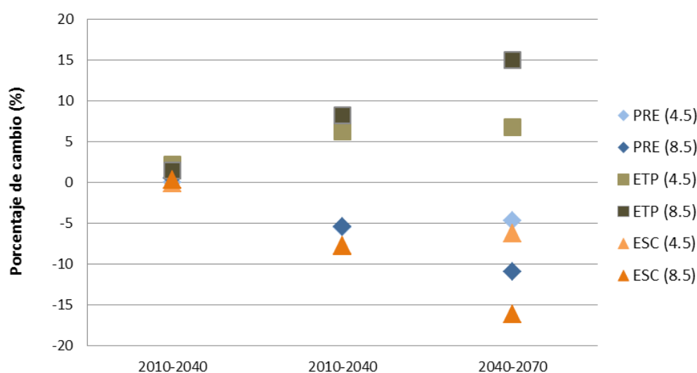
Figura 2: Representación gráfica de porcentaje de cambio con respecto al periodo control y escenarios RCP aplicados a la RNF del río Murias hasta la junta con el río Balouta para las variables de precipitación (PRE), evapotranspiración potencial (ETP) y escorrentía (ESC) con respecto al periodo de control. Fuente: Elaboración propia a partir de la aplicación informática CAMREC versión 1.0 (julio de 2017) desarrollada por el CEDEX.
