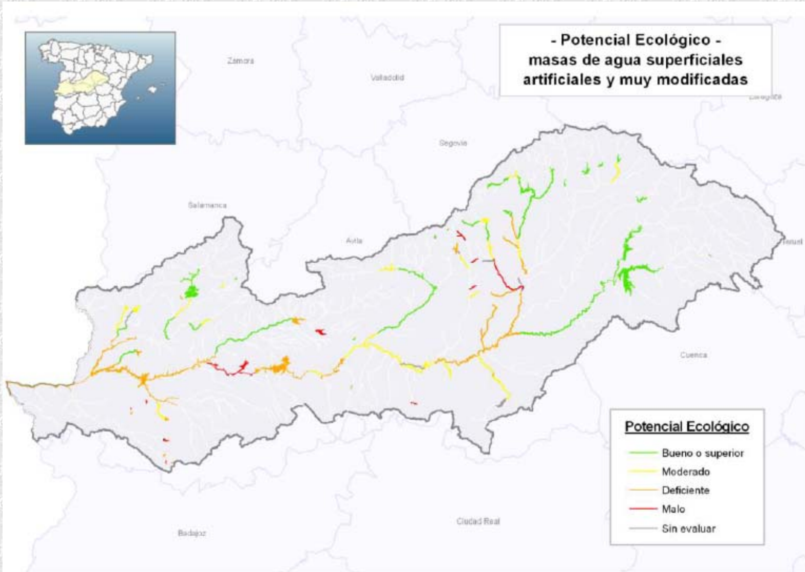
Figura 2. Potencial ecológico Masas de agua muy modificadas o artificiales
