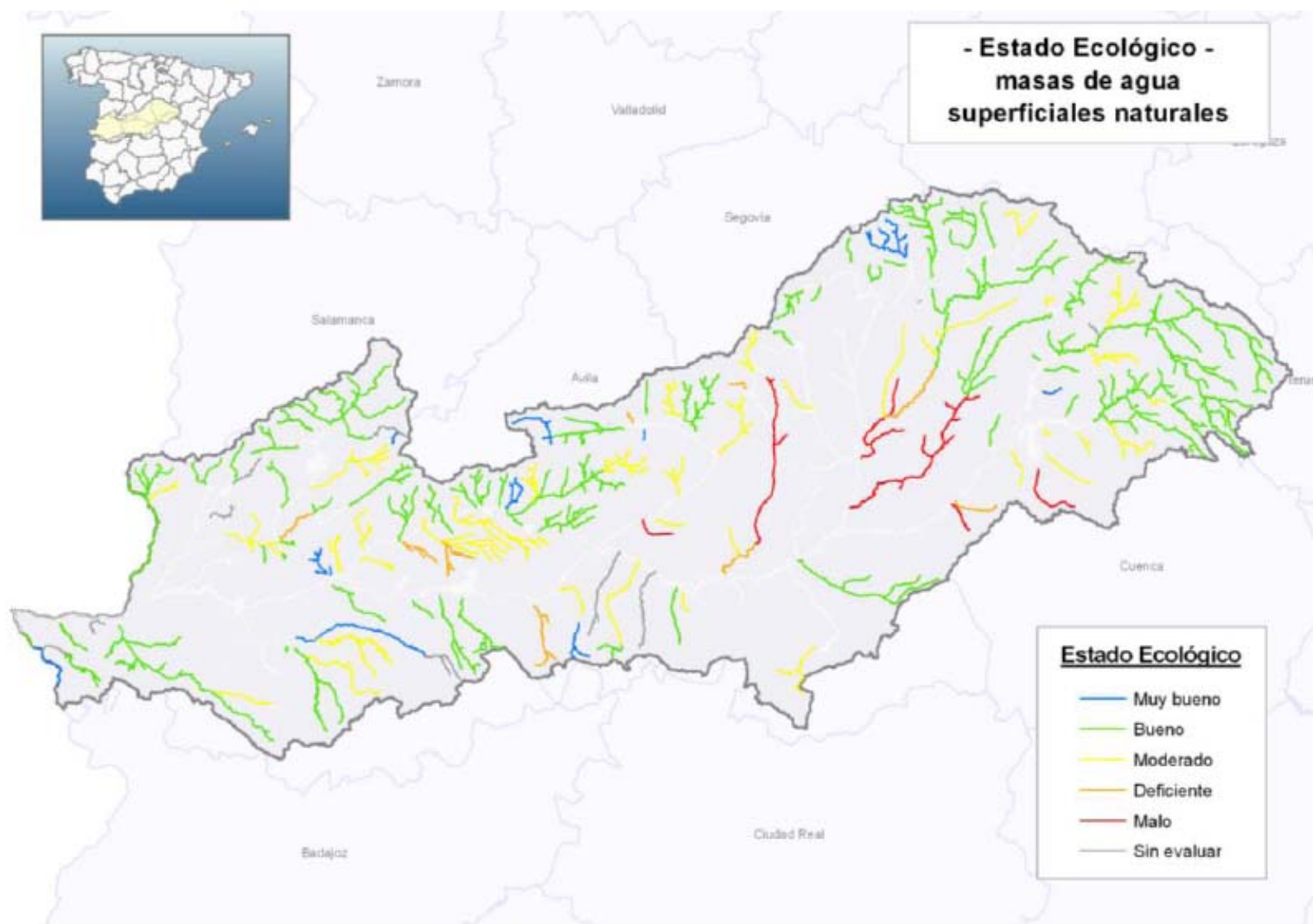
Figura 1. Estado ecológico masas de agua naturales de la cuenca del Tajo
